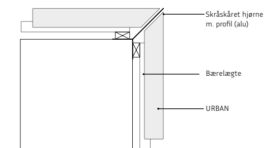
Skråskåret hjørne med afslutningsprofil
