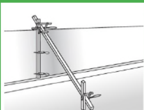
Figur 2. Metode 1. Murværk afstivet med en lodret og en skråtstillet planke hhv. fastgjort til mur og terræn.
