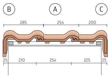
Montering af vindskedesten
